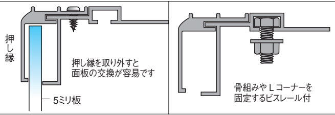
939304 看板枠 19 H 用 L コーナー
